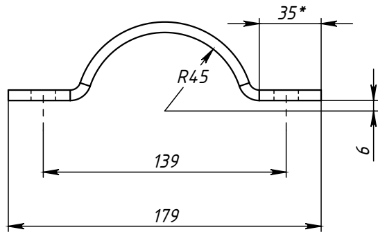
Поз.2 (Полухомут)
